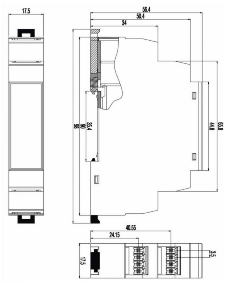
Obr. 3: Rozměry převodníku
